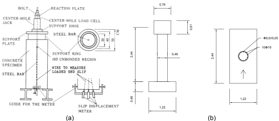
Figura 6: Dimensões gerais dos modelos SD30 [20] e Test 19 [5] testados experimentalmente.
