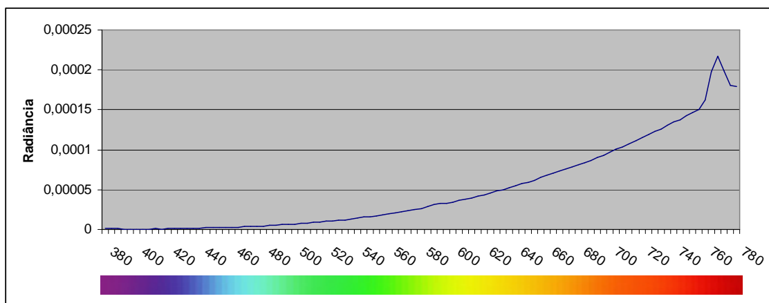
Gráfico 1: Valores de radiância medidos, na faixa visível ao olho humano do espectro electromagnético, com uma das amostras de azeite sem adição de sal
