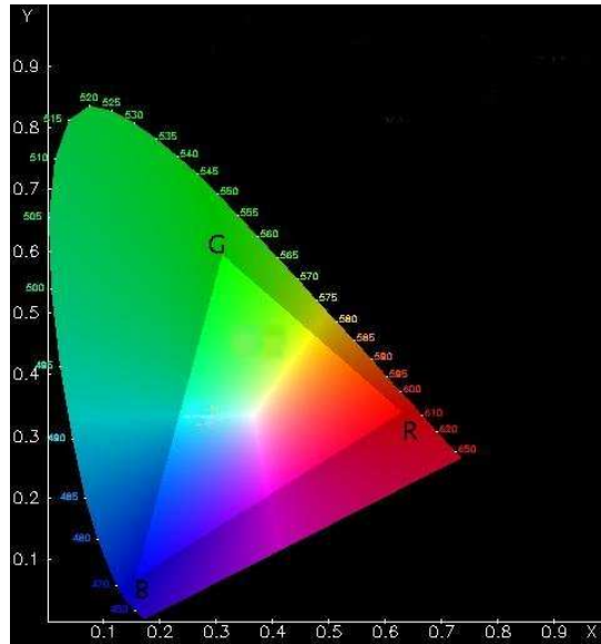
Figura 1: Diagrama de cromaticidade CIE, onde é perceptível a limitação cromática do RGB [Walter96]
