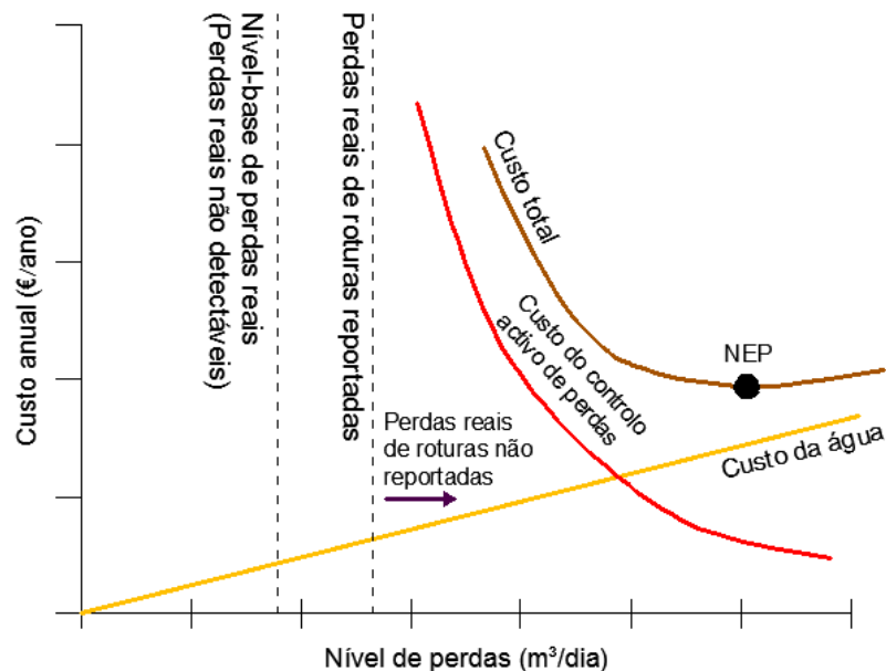
Figura 2.15 – Nível económico de perdas reais. Fonte: Alegre et al. (2005).
