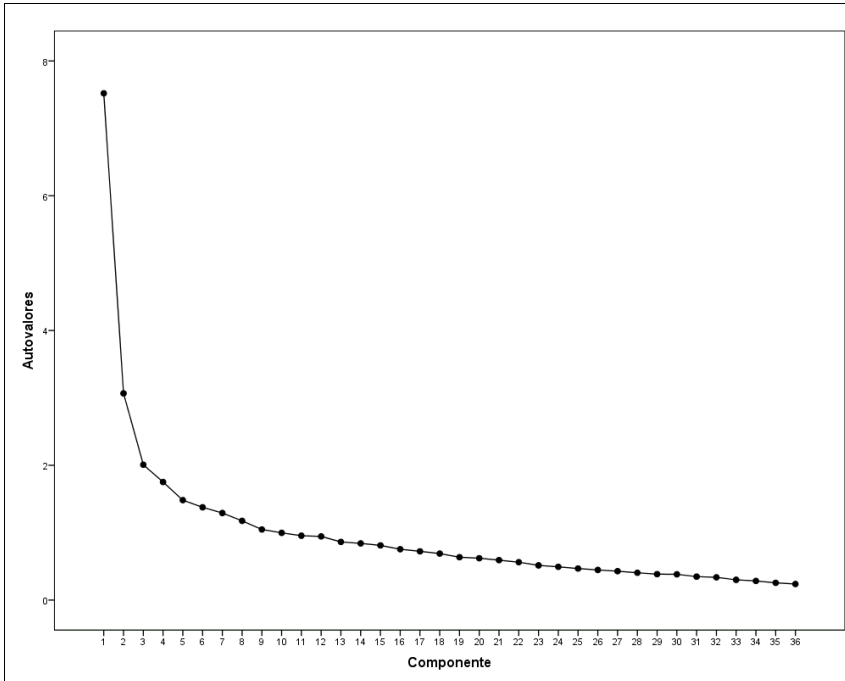
Figura 6 - Scree Plot dos Fatores Calculados
